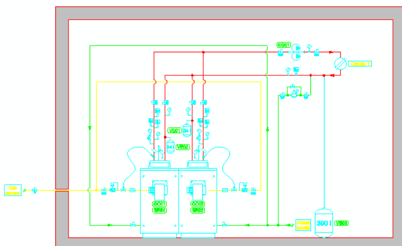
Figura 4.7 - Particolare dello schema di impianto
